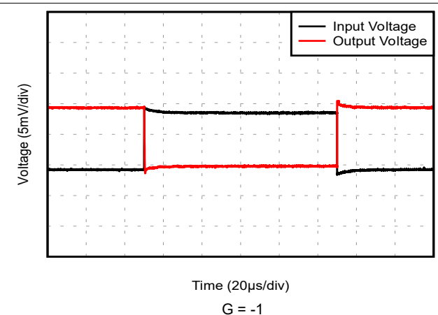
図 5-36. 小信号ステップ応答
