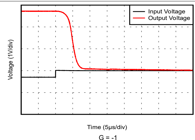
図 5-34. 過負荷回復
