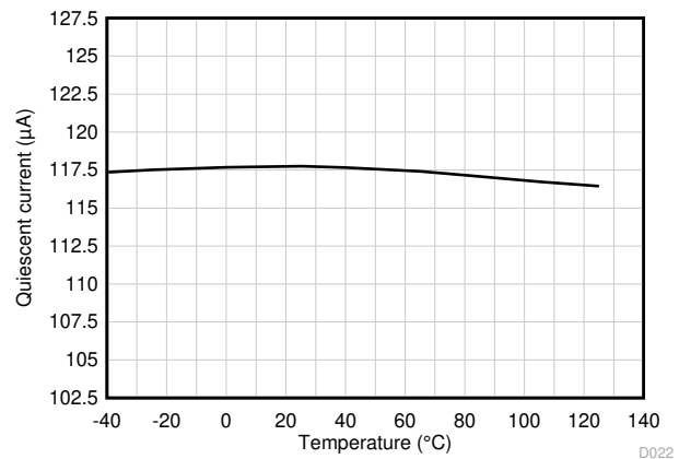
図 6-26. 静止電流と温度との関係
