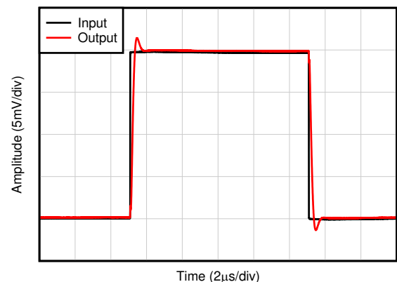
図 6-37. 正の過負荷からの回復
