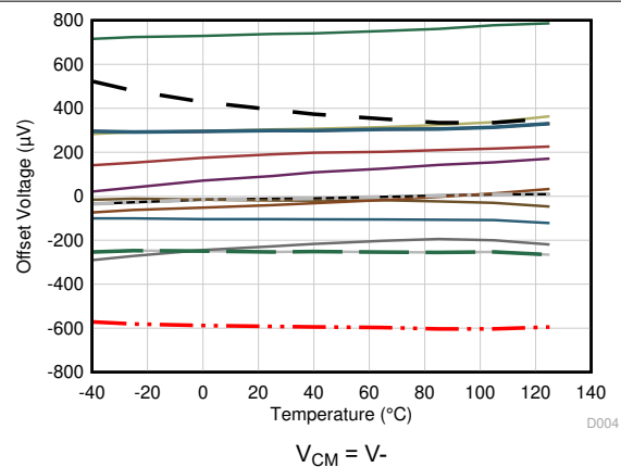
図 6-2. オフセット電圧ドリフトの分布
