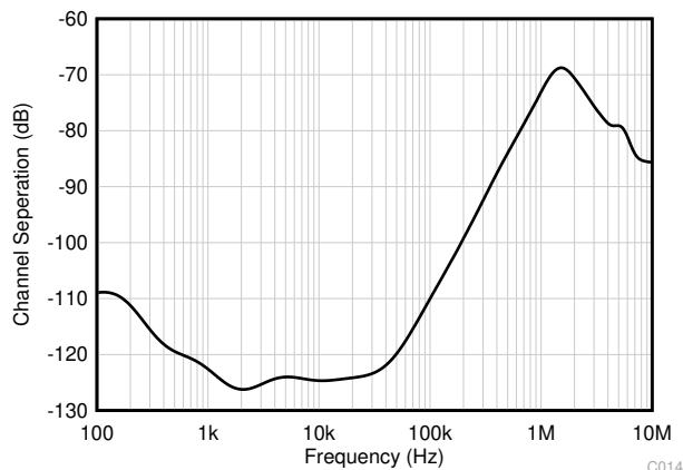
図 6-46. チャネル・セパレーションと周波数との関係
