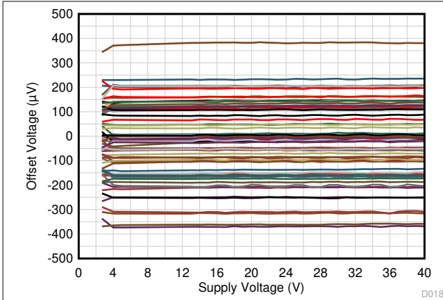
図 5-11. オフセット電圧と電源電圧との関係 74 個のアンプにおけるデータ
