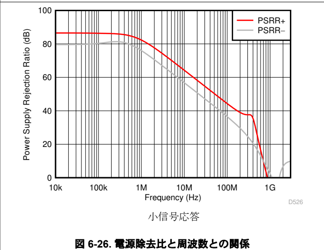
図 6-26. 電源除去比と周波数との関係
