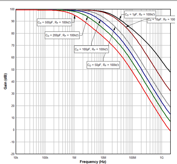
図 9-10. 3 フォトディテクタ入力特性 TIA 周波数応答
