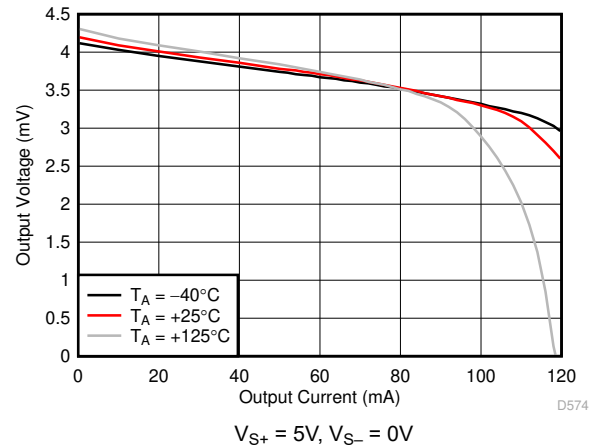
図 6-38. 出カスイングとソース電流との関係
