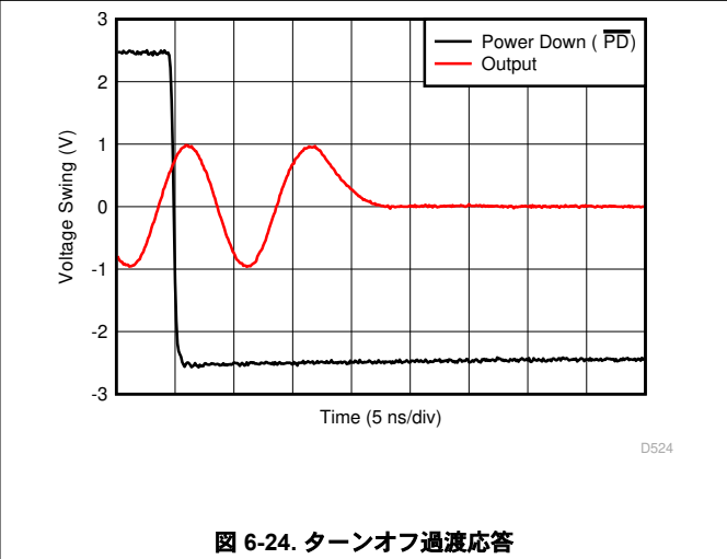
図 6-24. ターンオフ過渡応答
