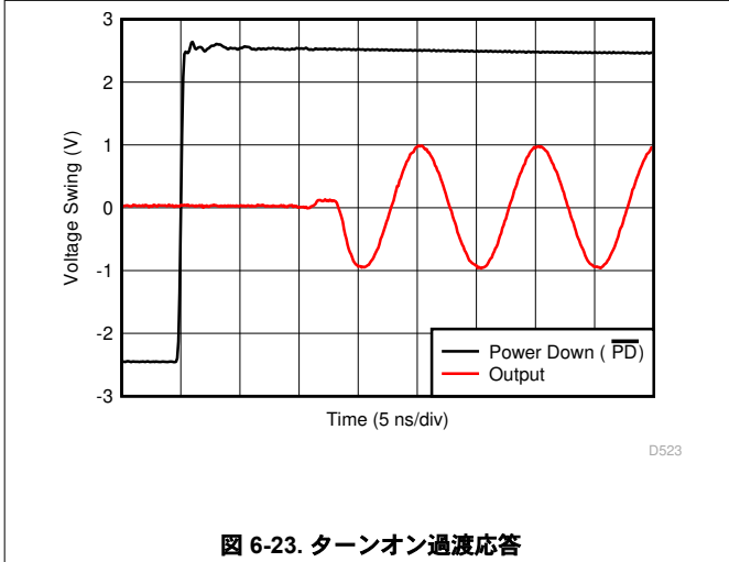
図 6-23. ターンオン過渡応答
