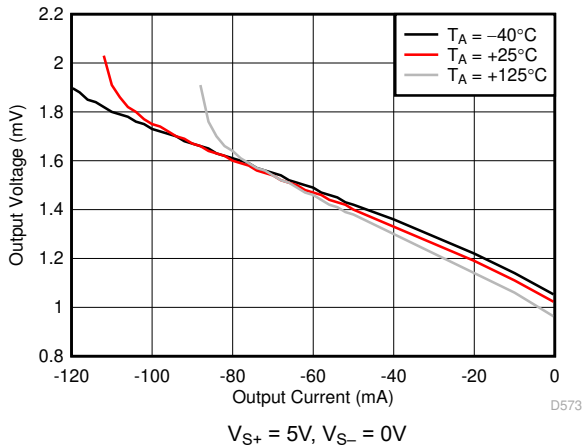
図 6-37. 出カスイングとシンク電流との関係
