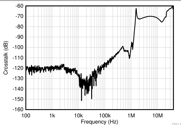
図 5-42. チャネル セパレーションと周波数との関係
