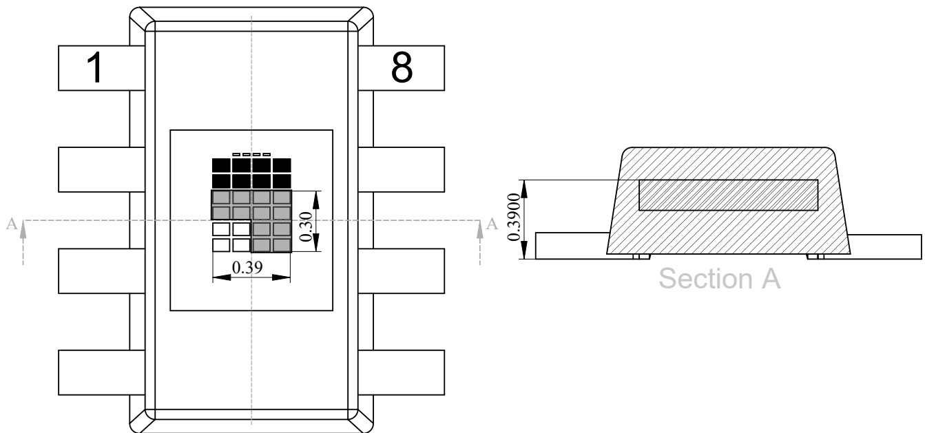
図 8-2. Sensor Position
