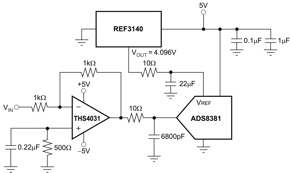
図 7-8. REF3140 は、ADS8381 を駆動するための高精度リファレンスを提供します
