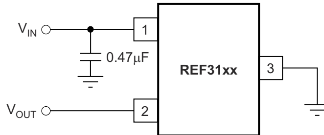
図 8-1. REF31xx の動作に必要な標準的接続
