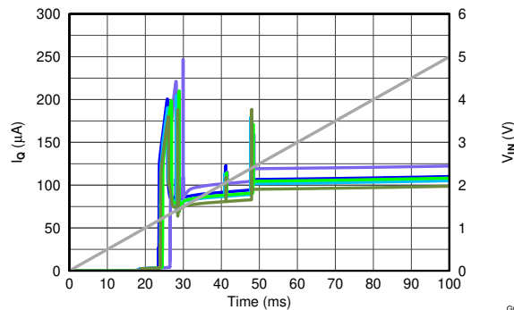
図 6-19. REF3125 のスタートアップ
