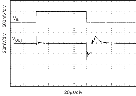
図 6-13. ライン過渡 C_L = 0\text{pF}
