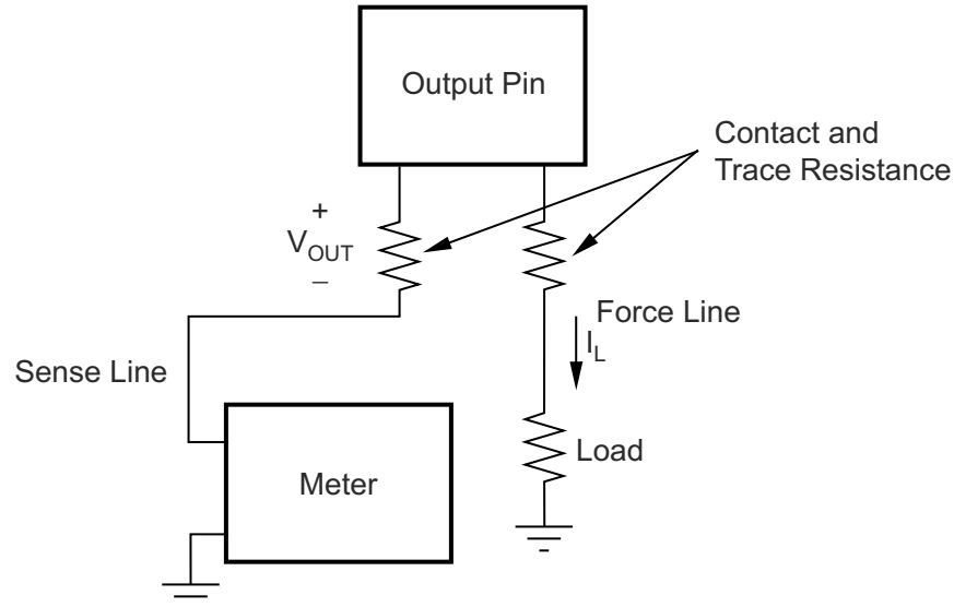
図 7-4. REF31xx の正確なロードレギュレーション
