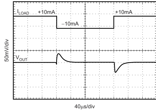
図 6-16. 負荷過渡 C_L = 1\mu\text{F} 、 \pm 10\text{mA} 出力パルス
