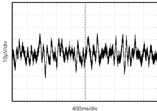
図 7-2. 0.1Hz~10Hz のノイズ
