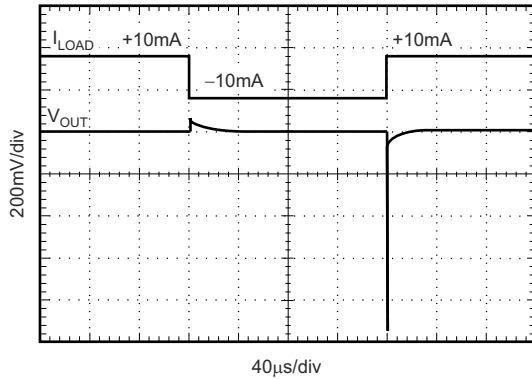
図 6-15. 負荷過渡 C_L = 0\text{pF} 、 \pm 10\text{mA} 出力パルス
