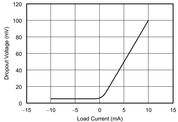
図 6-4. ドロップアウト電圧と負荷電流との関係
