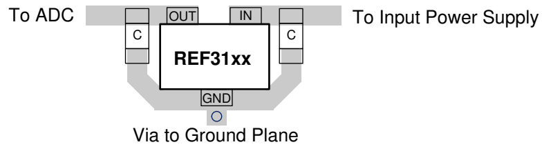
図 8-6. レイアウト例
