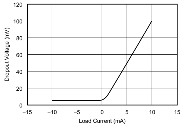
ドロップアウト電圧と負荷電流との関係
