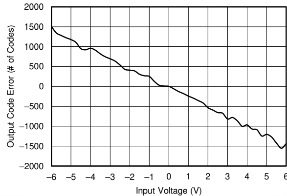
図 8-5. 出力コード誤差と基準電圧との関係
