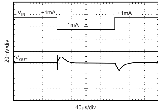
図 6-18. 負荷過渡 C_L = 1\mu\text{F} 、 \pm 1\text{mA} 出力パルス
