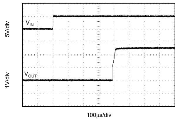
図 6-10. ステップ応答、 C_L = 0 、5V スタートアップ
