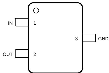
図 5-1. DBZ パッケージ 3 ピン SOT-23 上面図
