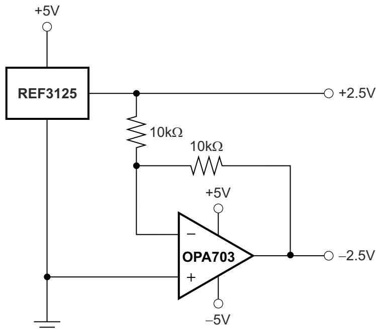
図 7-5. REF3125 と OPA703 を組み合わせて正および負の基準電圧を生成
