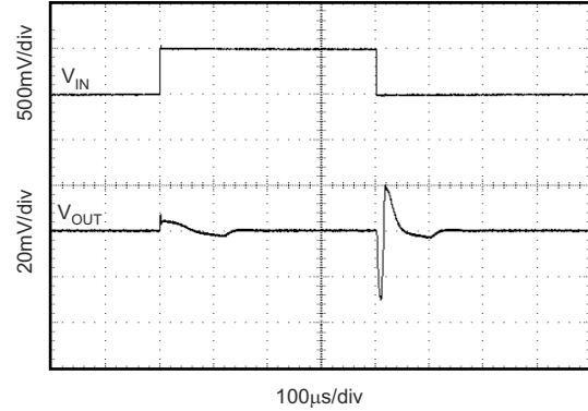
図 6-14. ライン過渡 C_L = 10\mu\text{F}
