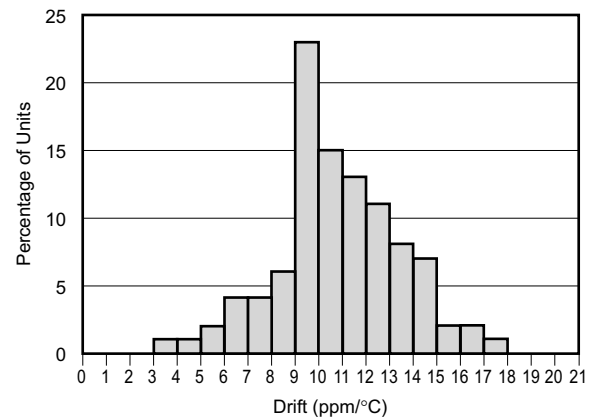
図 6-2. 温度ドリフト (-40°C ~ +125°C)
