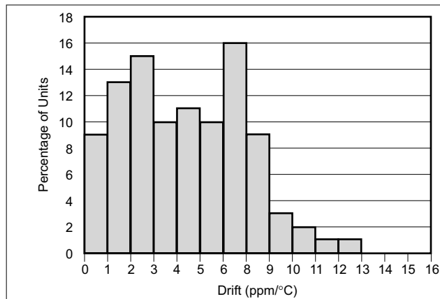
図 6-1. 温度ドリフト (0°C ~ 70°C)
