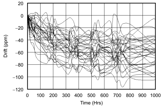
図 6-12. REF3112 長期安定性
