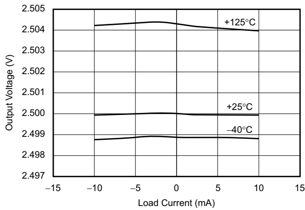
図 6-9. 出力電圧 対 負荷電流
