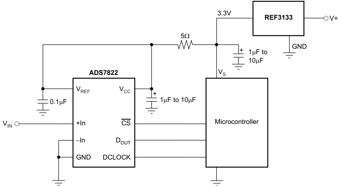
図 7-6. 基本的なデータ収集システム 1
