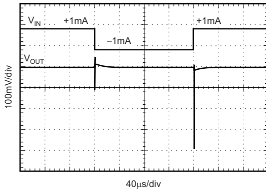
図 6-17. 負荷過渡 C_L = 0\text{pF} 、 \pm 1\text{mA} 出力パルス
