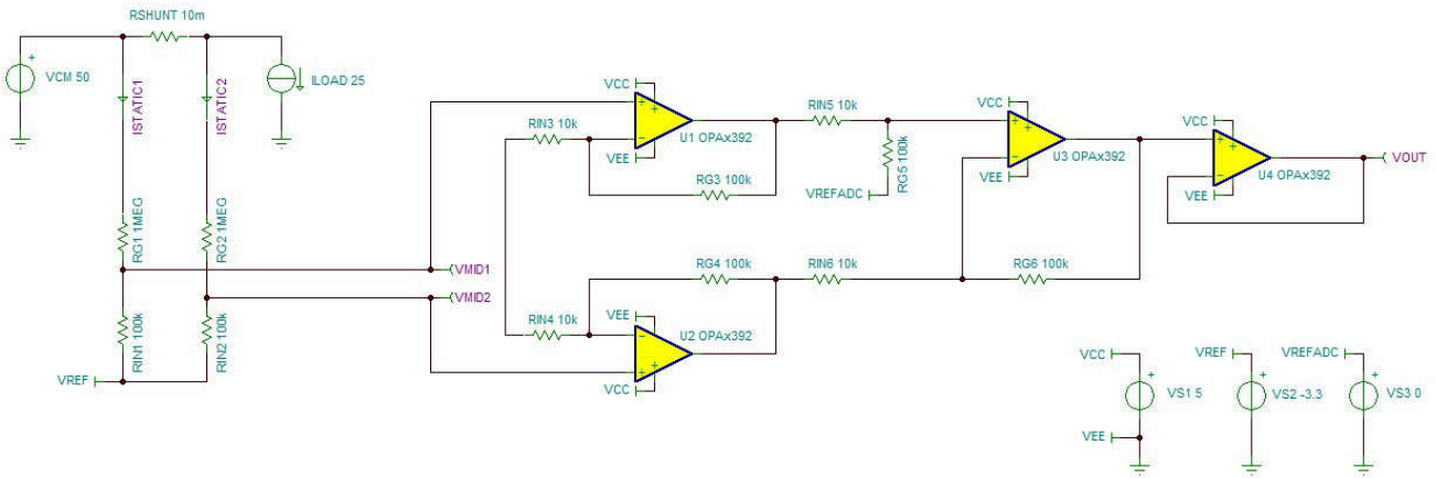
図 8-16. TINA-TI の回路モデル
