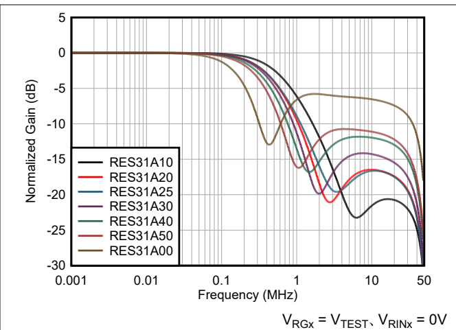
図 5-38. 帯域幅と周波数との関係、 R_{Gx}
