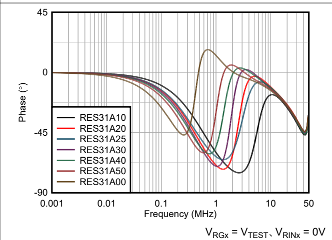
図 5-40. 位相と周波数との関係、 R_{Gx}
