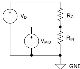
図 6-3. 分圧回路
