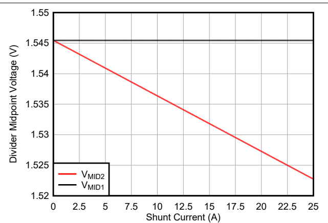
図 8-18. V_{MID} のシミュレーション結果
