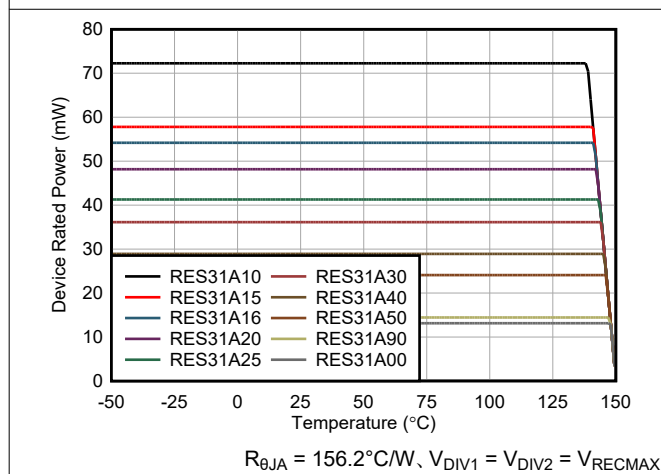
図 5-35. デバイス定格電力と周囲温度との関係
