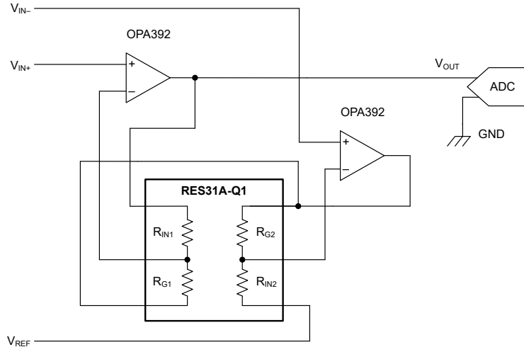
図 8-8. RES31A-Q1 を使用する、差動入力、シングルエンド出力の計測アンプ
