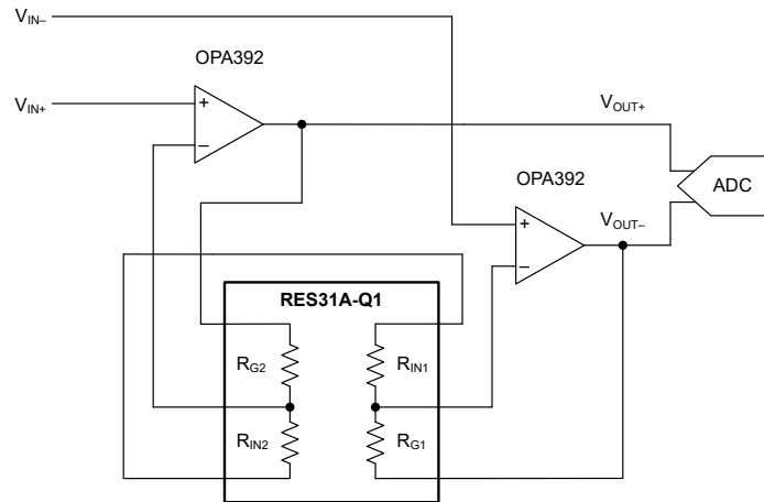
図 8-7. RES31A-Q1 を使用する差動入力、差動出力の計測アンプ
