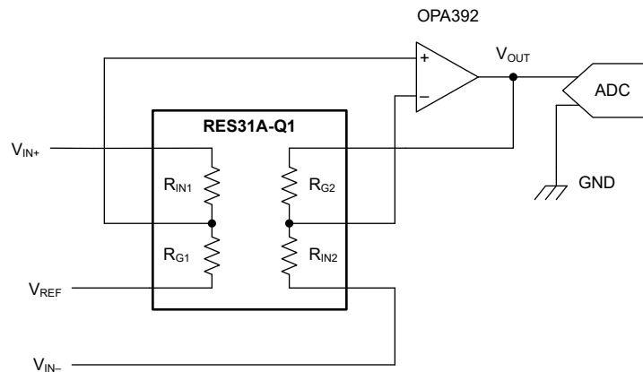
図 8-6. RES31A-Q1 を使用したディスクリット差動アンプ
