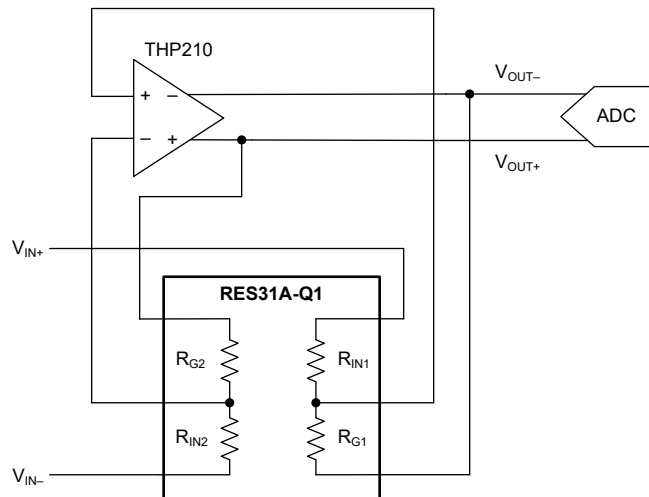
図 8-9. RES31A-Q1 を使用した完全差動アンプのゲイン設定
