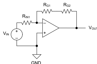
図 8-13. V_{OUT} = -20 \times V_{IN} 、RES31A00-Q1 で実装
