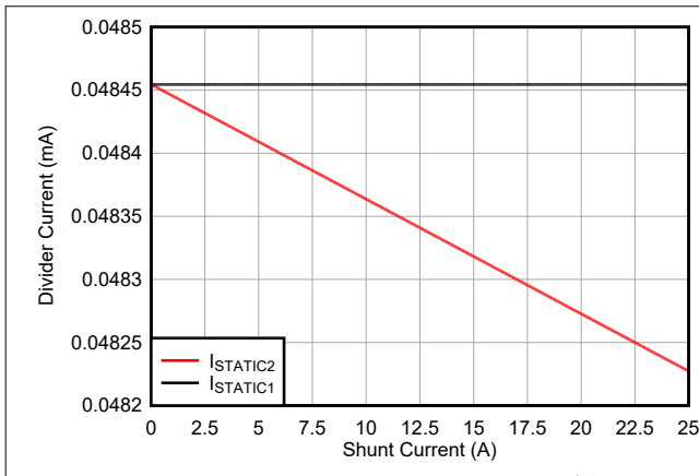
図 8-17. I_{STATIC} のシミュレーション結果
