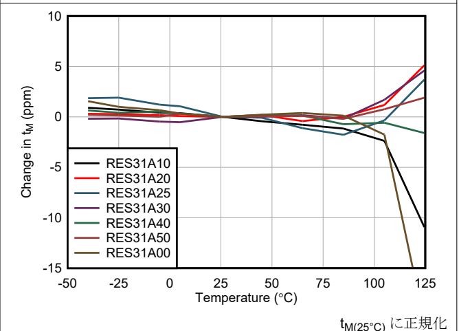
図 5-24. t_M と温度との関係
