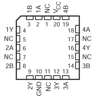
NC – No internal connection 図 3-2. SN54AC32 FK パッケージ、 14-ピン LCCC (上面図)
