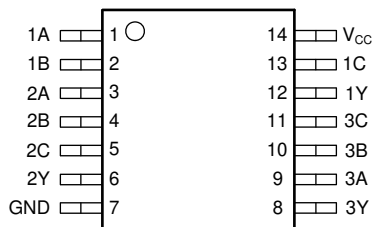
図 4-1. J または W パッケージ (上面図)
