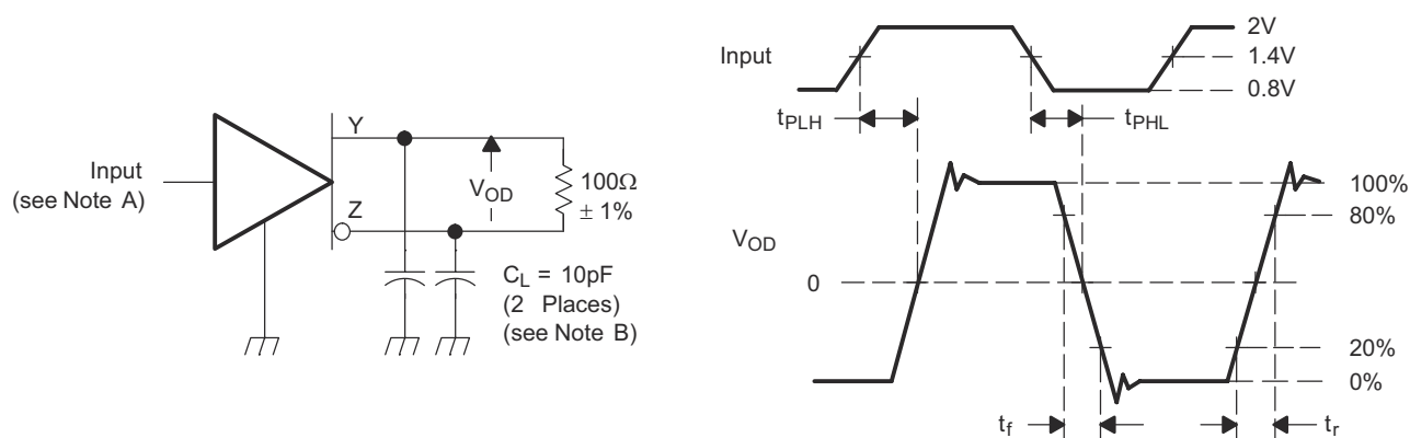
図 6-1. 電圧および電流の定義
