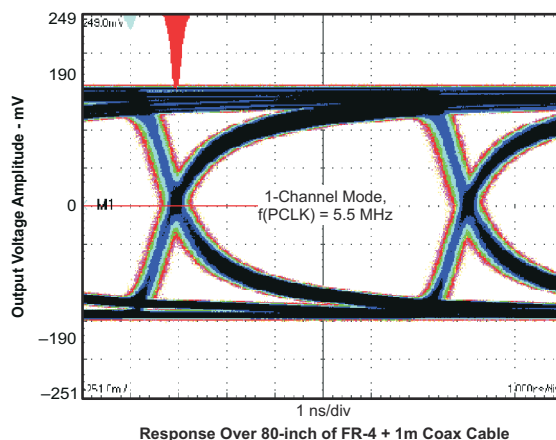
図 9-10. QVGA Output Waveform
