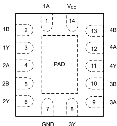
図 4-1. SN74AC09 BQA または パッケージ (上面図)
