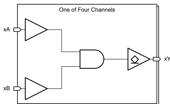
概略回路図
