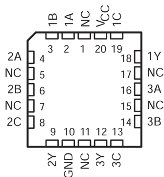
図 4-2. SN54AC10 FK パッケージ (上面図)
