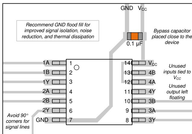
図 7-1. SN74AC86 のレイアウト例
