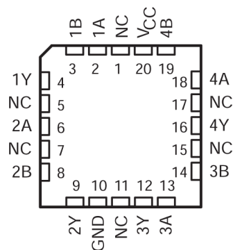
図 3-2. SN54AC86 FK パッケージ (上面図)
