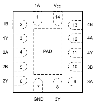
図 3-3. BQA パッケージ (上面図)
