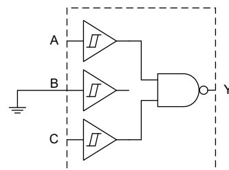
2 入力 NAND ゲート
