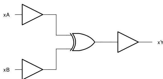
ロジック図
