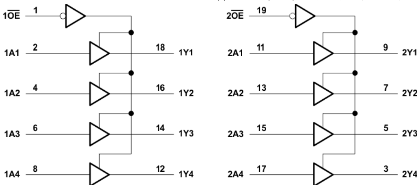
概略回路図
