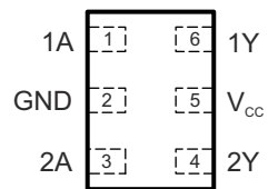
図 4-3. DSF パッケージ 6 ピン X2SON 上面図
