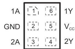
図 4-2. DRY パッケージ 6 ピン USON 上面図
