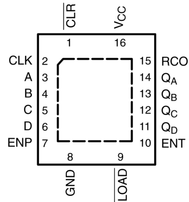
図 3-2. SN74LV163A RGY パッケージ、16 ピン VQFN (上面図)
