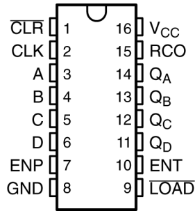
図 3-1. SN74LV163A D、DB、DGV、NS、PW パッケージ、16 ピン SOIC、SSOP、TVSOP、SOP、TSSOP (上面図)
