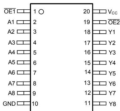
図 4-2. SN74LV8T540 PW、DGS パッケージ (上面図)
