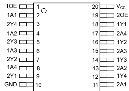
図 4-2. SN74LVC241A PW、DGS パッケージ (上面図)
