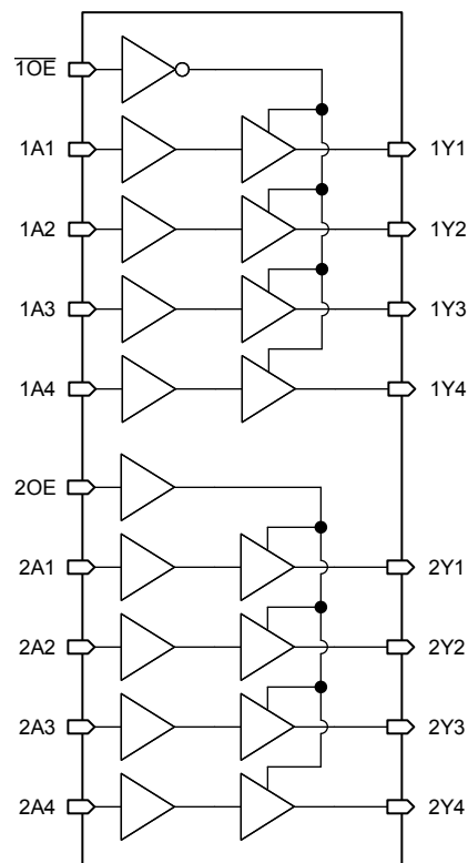
図 7-1. 論理図 (正論理)
