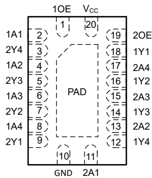
図 4-1. SN74LVC241A RKS パッケージ (上面図)
