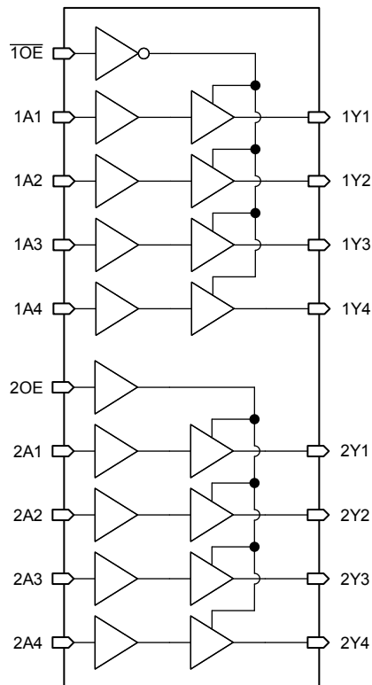
機能ブロック図
