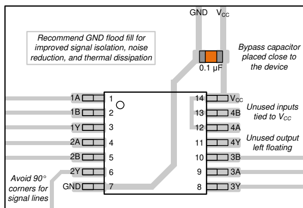
図 8-3. Example Layout for the SN74LVC7032A-Q1
