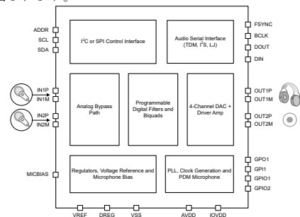
概略ブロック図
