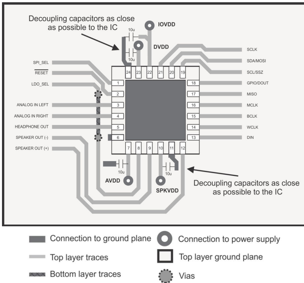
図 9-5. Layout Diagram
