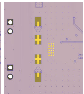
Bot Layer Layout
