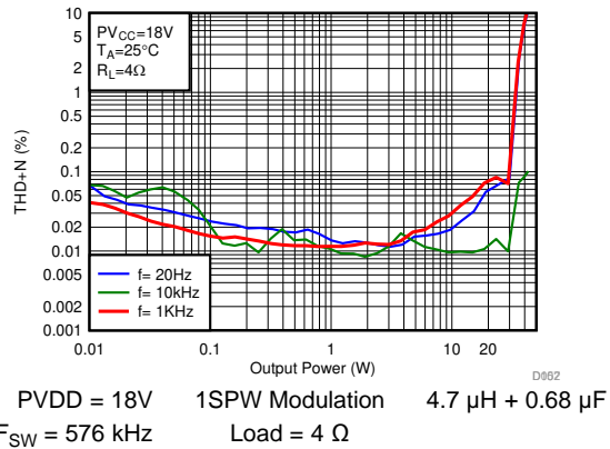
图 49. THD+N vs Output Power
