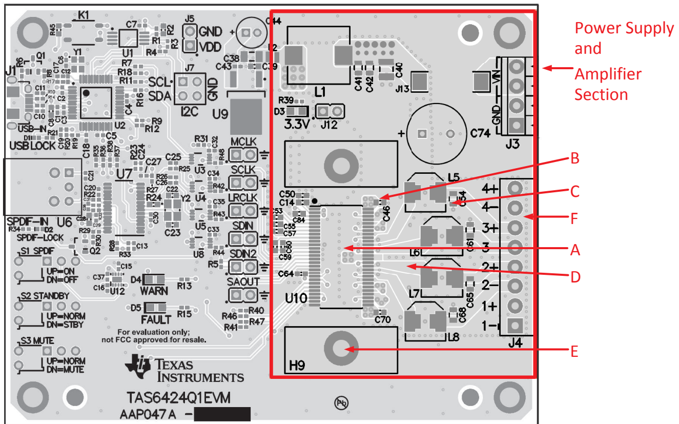
图 85. EVM Layout
