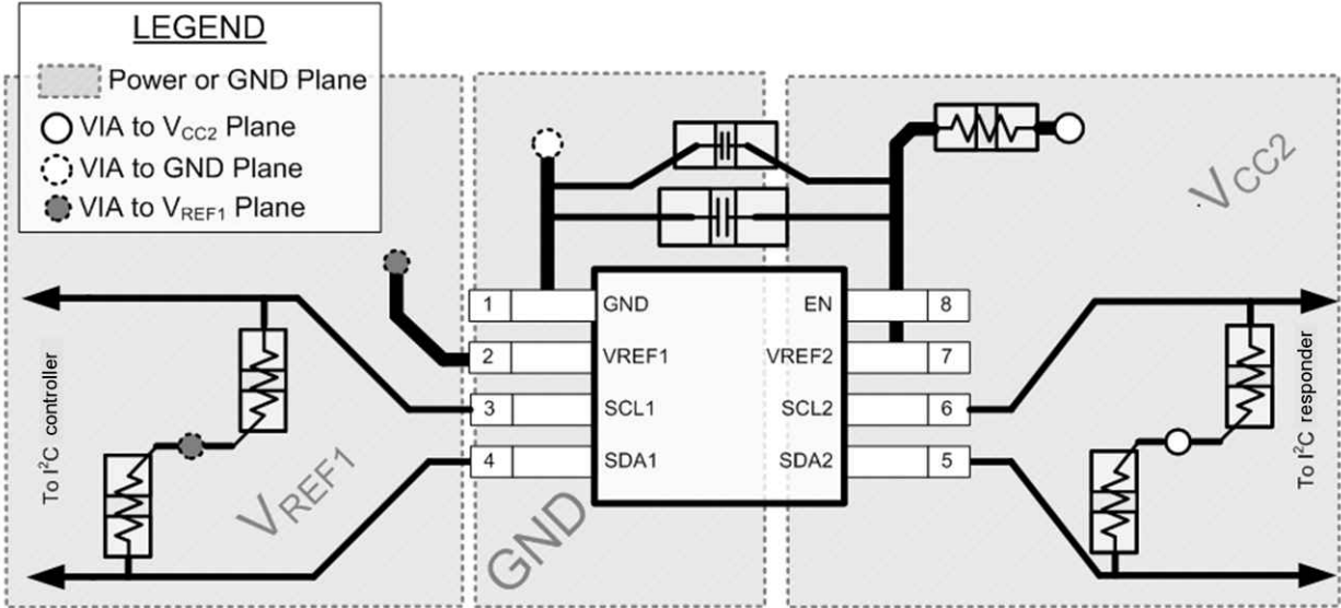
图 9-8. Layout Example
