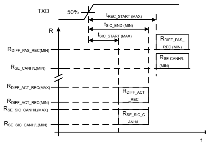
図 6-13. アクティブおよびパッシブ リセシップ位相時の SIC タイミングとインピーダンス
