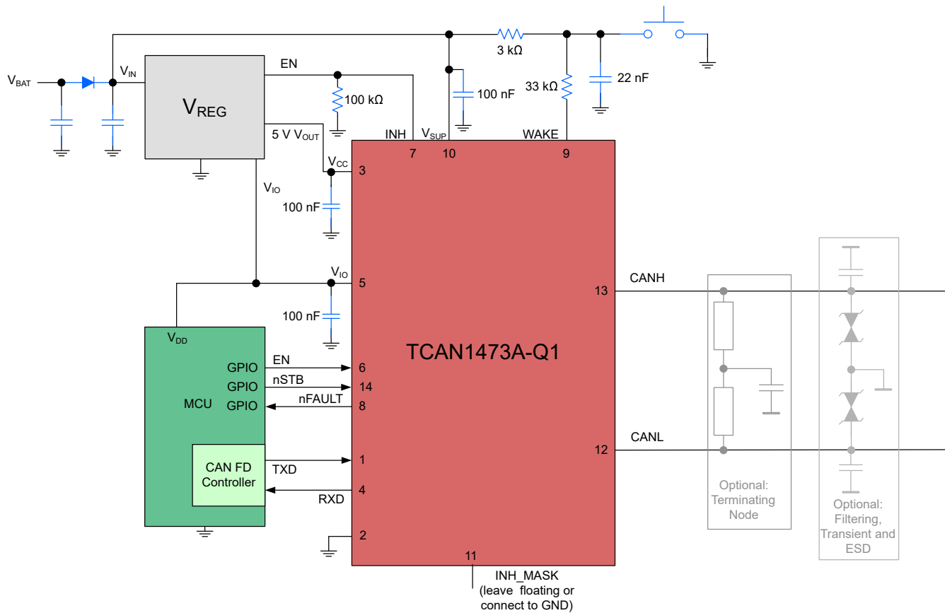
概略回路図
