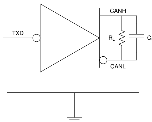
図 6-3. 電源テスト回路
