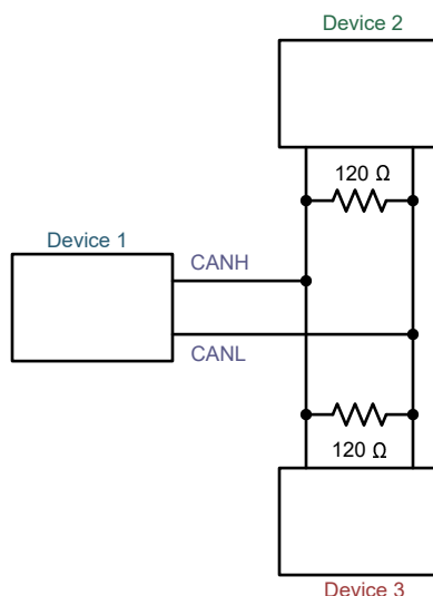
図 8-47. 3 ノードの例
