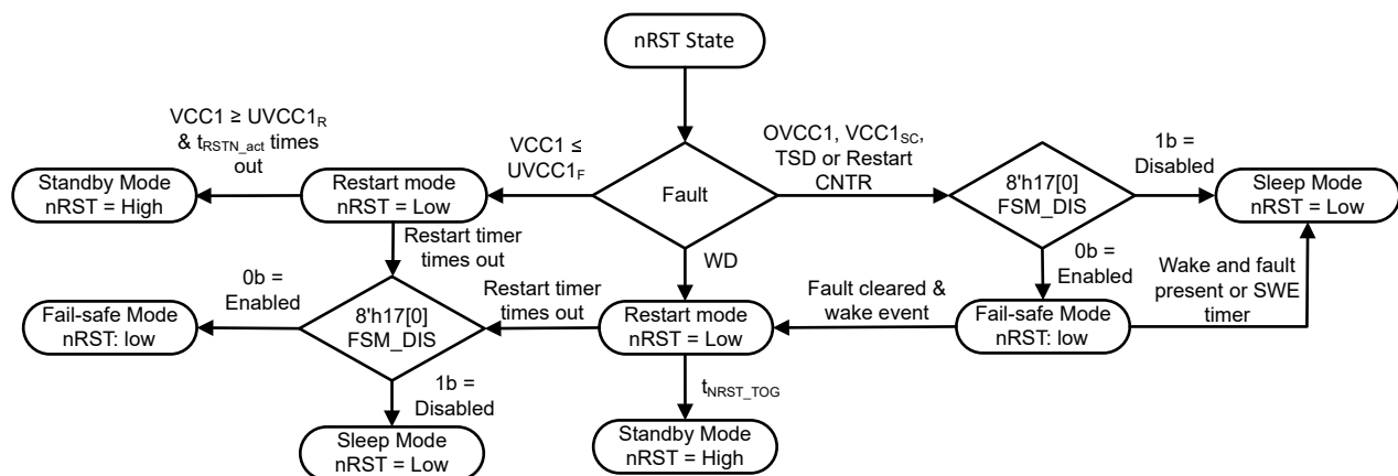
図 8-7. nRST 状態図
