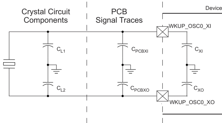
図 6-27. 負荷容量
