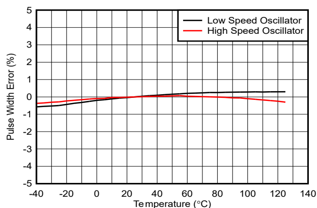
図 5-3. パルス幅誤差と温度との関係
