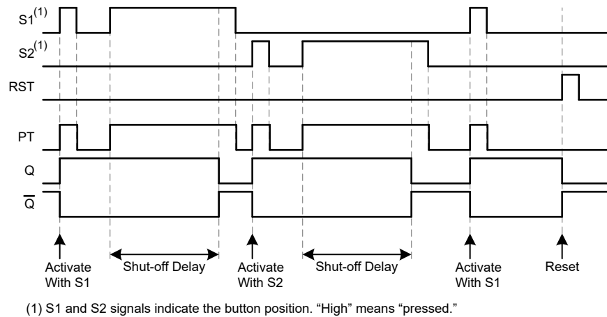
図 8-2. 出力タイミング図
