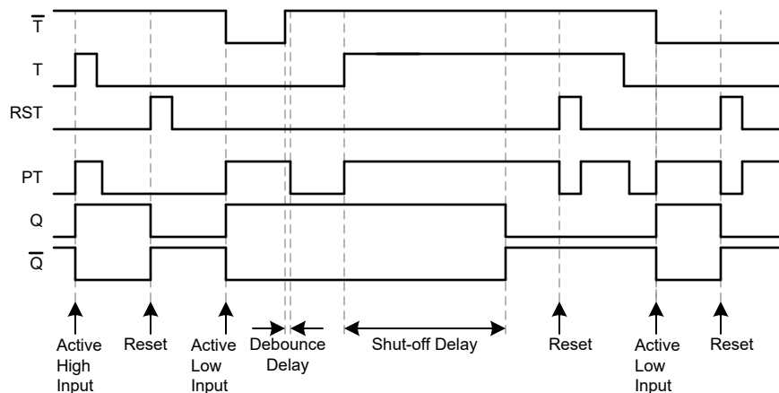
図 5-1. タイミング図
