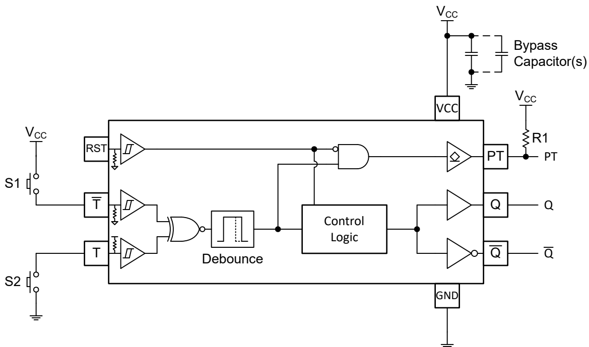
図 8-1. TDEL1G533 を使用したモーメンタリ スイッチ インターフェイスの回路図
