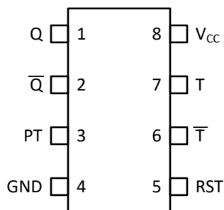
図 4-1. TDEL1G533 DRL パッケージ（上面図）
