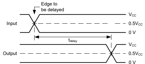
図 6-6. 電圧波形、エッジ遅延時間
