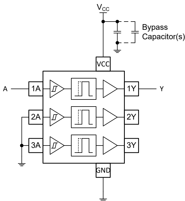
図 8-1. TDEL3G511 を使用した立ち上がりエッジ遅延回路図
