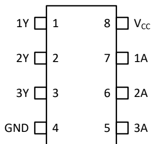
図 4-1. TDEL3G511 DRL パッケージ（上面図）
