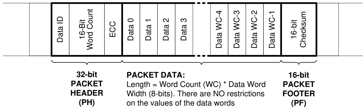
☒ 7-10. CSI-2 Long Packet Structure
