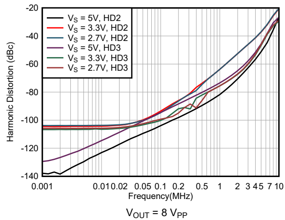
図 6-27. 高調波歪みと周波数との関係
