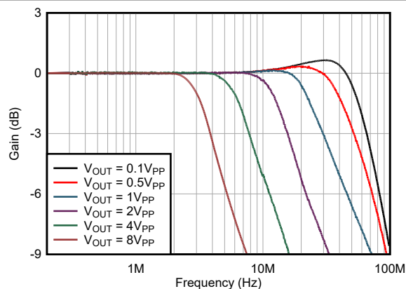
図 6-6. 大信号帯域幅と出力振幅との関係
