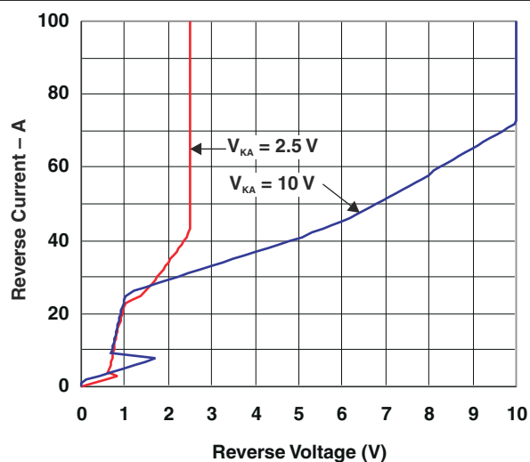
図 5-3. 逆特性と最小動作電流
