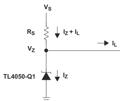
図 7-3. シャントレギュレータ
