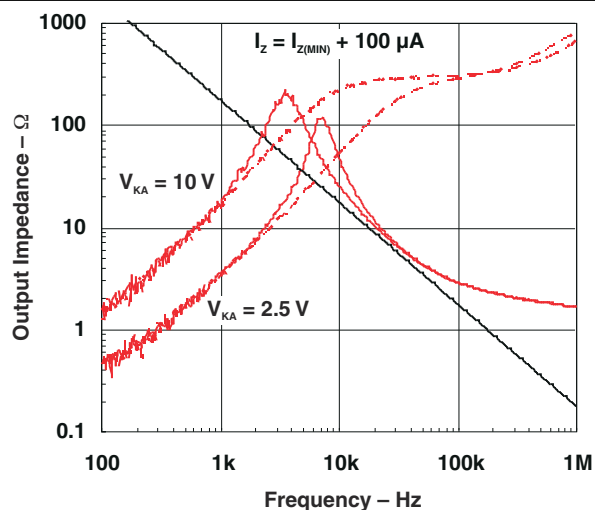
図 5-1. 出力インピーダンス対周波数
