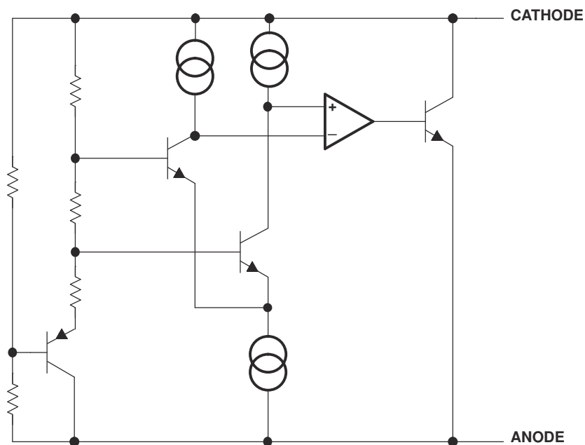
図 6-1. 機能ブロック図
