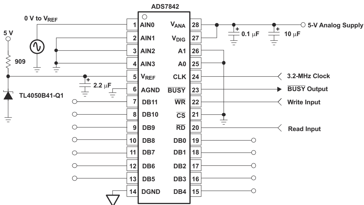
図 7-2. TL4050x41-Q1 を使用したデータ アクイジション回路
