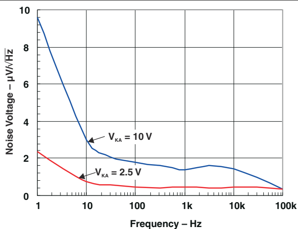
図 5-4. ノイズ電圧と周波数との関係
