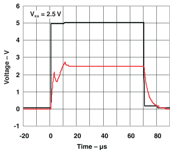
図 5-5. 大信号パルス応答
