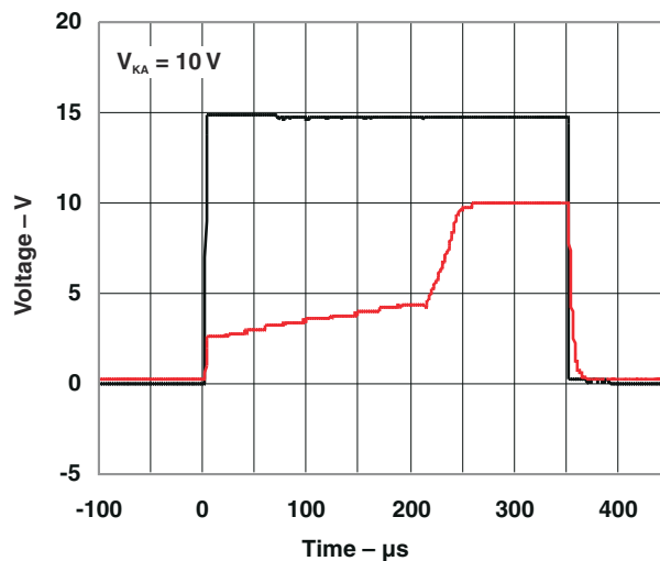
図 5-6. 大信号パルス応答
