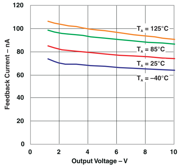
図 5-11. フィードバック電流と出力電圧との関係
