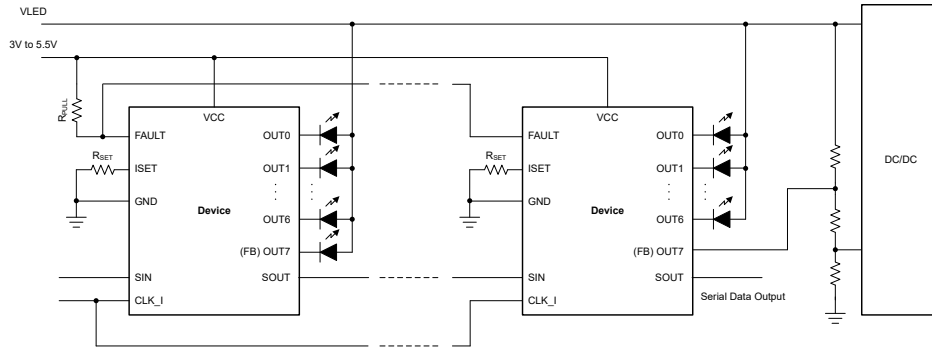
概略回路図
