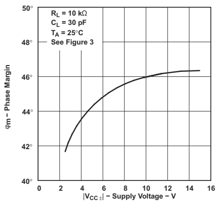
図 6-47. TLE2021 の位相マージンと電源電圧との関係
