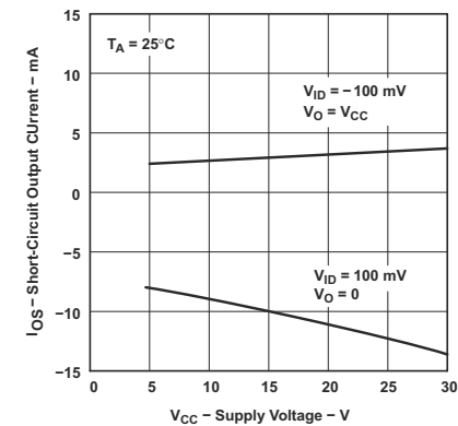
図 5-27. TLE2022xM および TLE2024xM 短絡出力電流と電源電圧との関係
