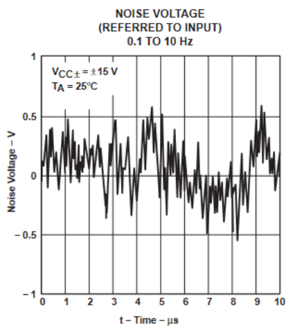
図 5-11. ノイズ電圧
