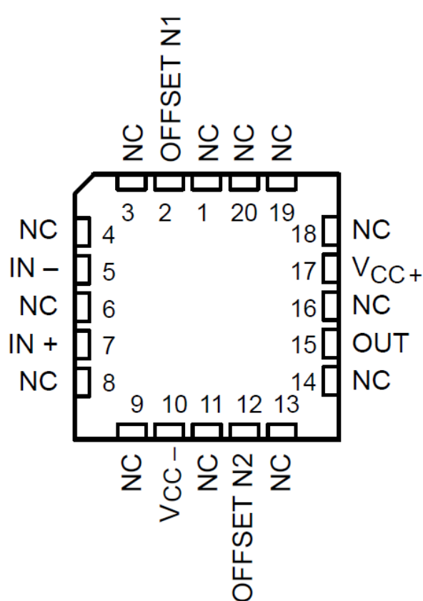
図 4-5. TLE2061M、TLE2061AM、TLE2061BM FK パッケージ (上面図)
