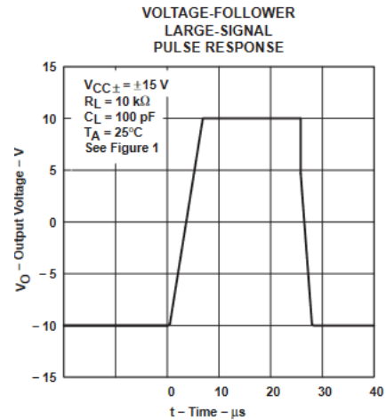
図 5-10. 電圧フォロワの大信号パルス応答
