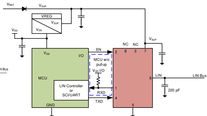
概略回路図、レスポンド・モード
