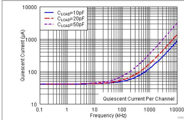
図 6-13. 電源電流と入力スイッチング周波数との関係
