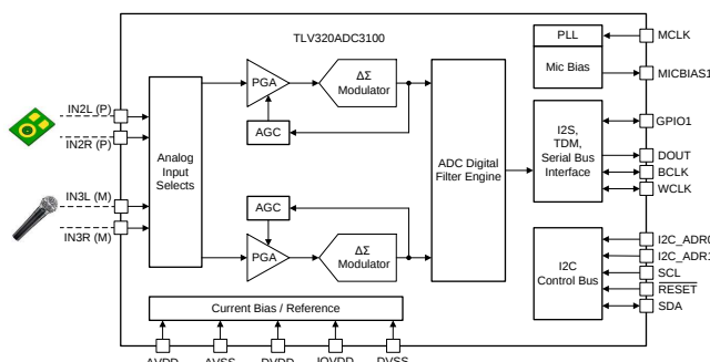
機能ブロック図
