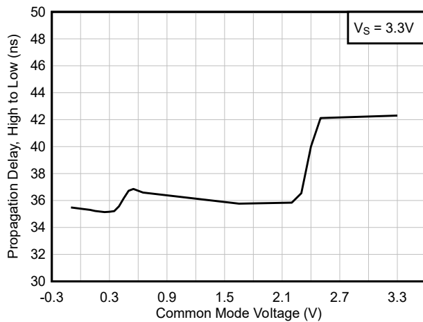
図 5-39. 伝搬遅延 - High から Low vs.3.3V でのコモンモード
