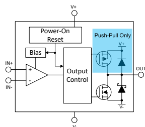
ブロック図
