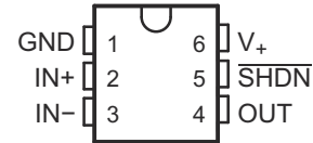
図 4-1. TLV341 DBV または DCK パッケージ、6 ピン 図 4-2. TLV341 DRL パッケージ、6 ピン SOT (上面図) SOT-23 または SC70 (上面図)
