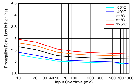
伝搬遅延 (Low から High) と入力オーバードライブ、5V
