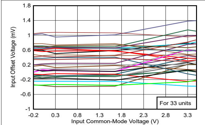
图 5-7. Offset vs. Common-Mode, 3.3V
