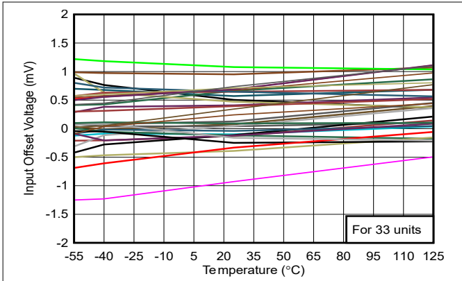
图 5-3. Offset vs. Temperature
