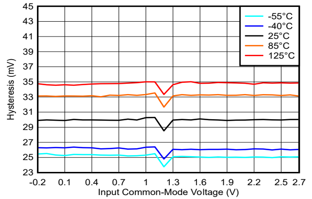
图 5-6. Hysteresis vs. Common-Mode, 2.5V
