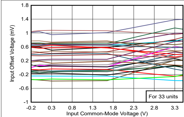
图 5-7. Offset vs. Common-Mode, 3.3V
