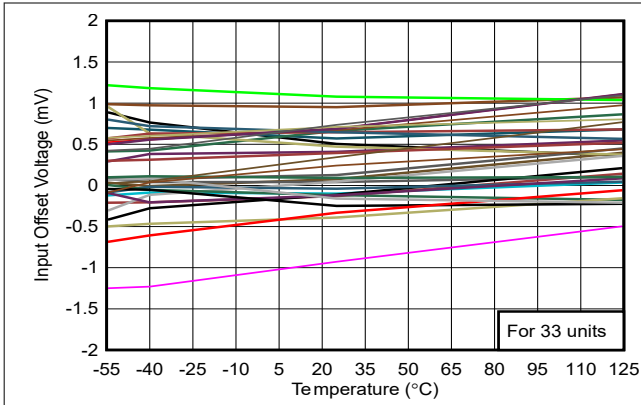
图 5-3. Offset vs. Temperature
