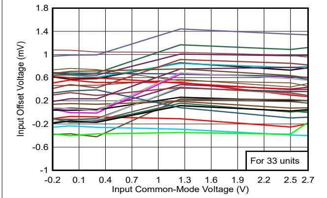
图 5-5. Offset vs. Common-Mode, 2.5V
