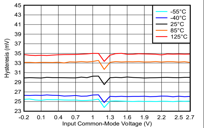
图 5-6. Hysteresis vs. Common-Mode, 2.5V
