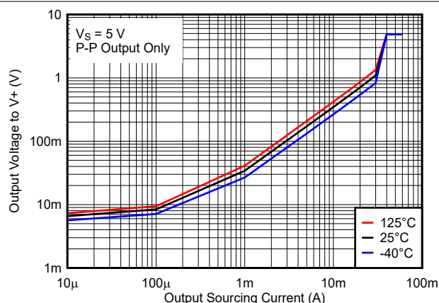
図 5-4. 出力電圧と出力ソース電流の関係、5V
