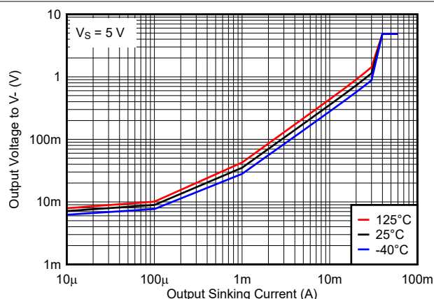
図 5-3. 出力電圧と出力シンク電流の関係、5V
