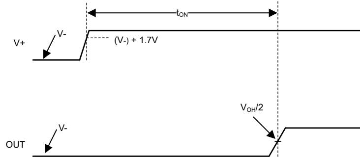
図 6-1. パワーオン リセットのタイミング図
