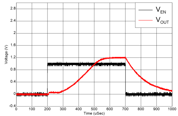
図 5-16. スタートアップ
