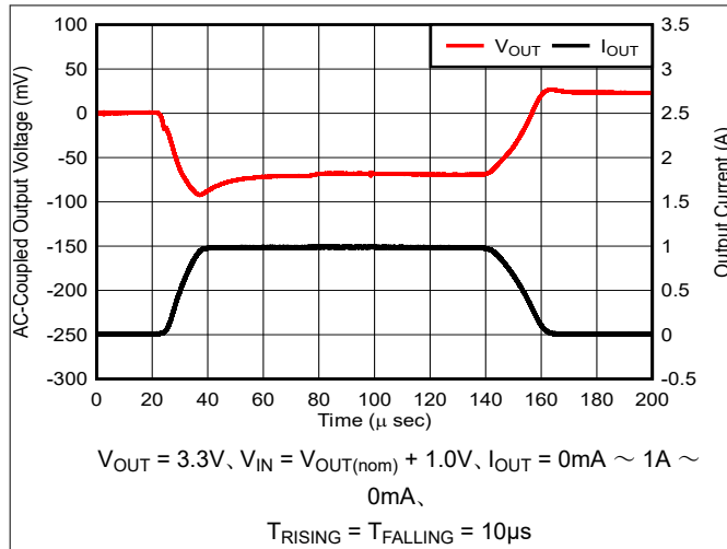
図 5-13. 負荷過渡
