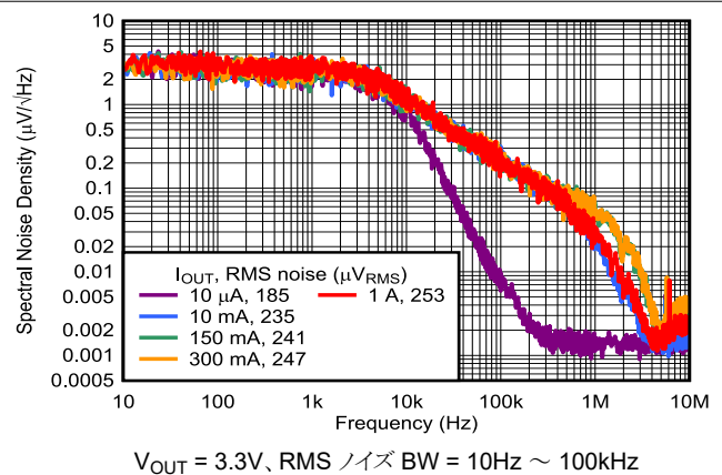
図 5-18. ノイズ
