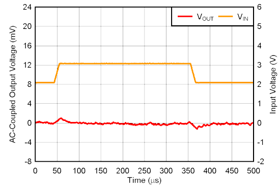
図 5-14. ライン トランジェント
