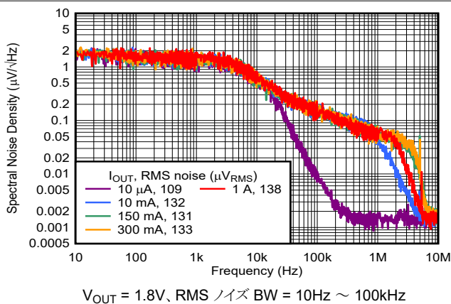
図 5-17. ノイズ
